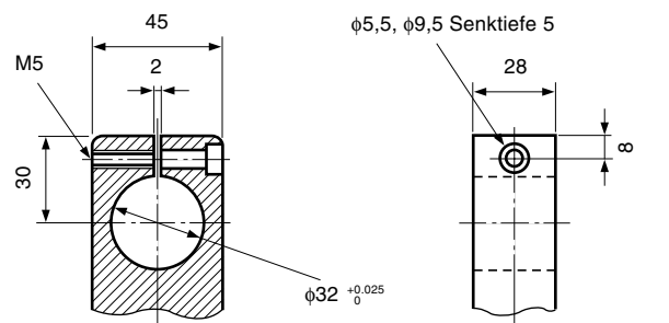
Anzugsmoment: 6 N•m Innensechskantschraube M5 verwenden.
